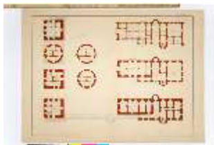
LIIMus.IV, Grundrisse, Neuschwanstein, Turm und Palas, Inv.-Nr. 1775e, DI009284, BSV-
